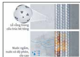
Hiện tượng cốt thép bị ăn mòn trong bê tông
